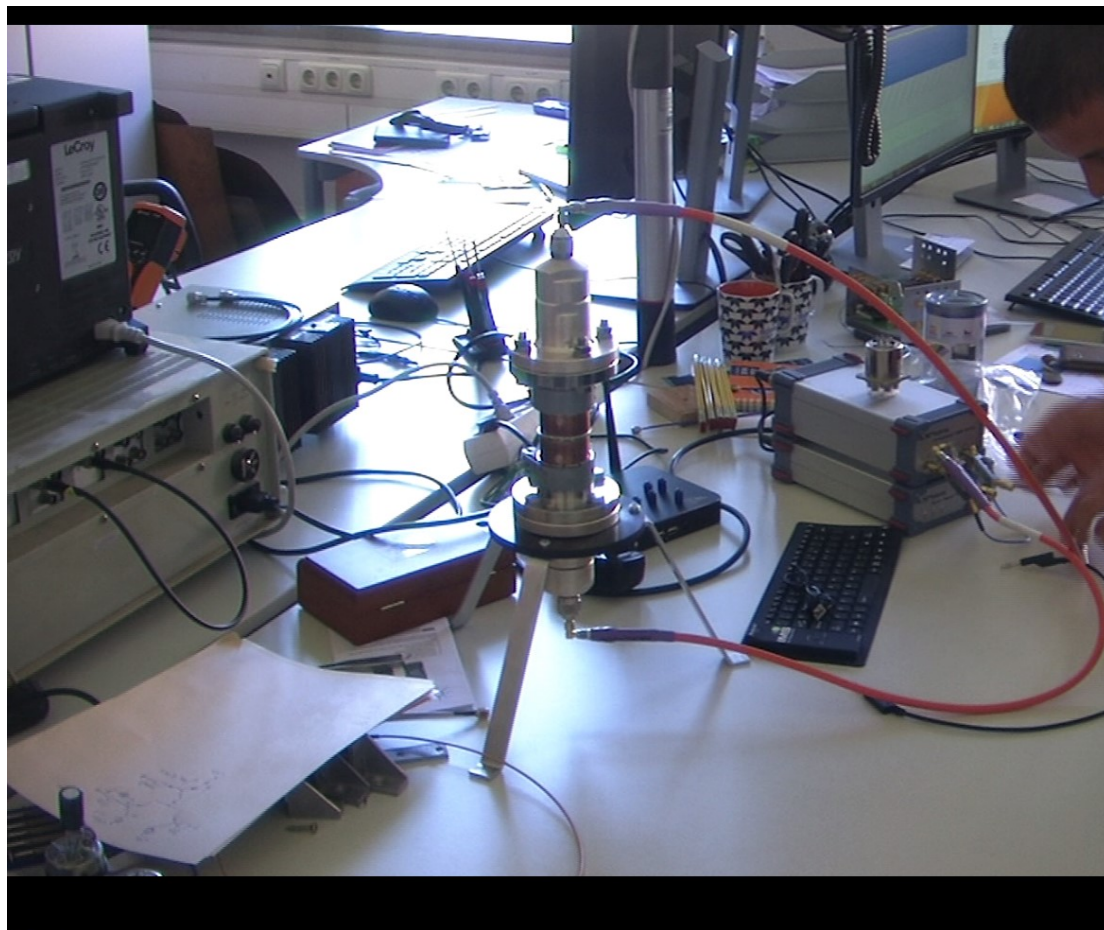
Ilmenau – Univerzita – Sonda na meranie výbušných látok
